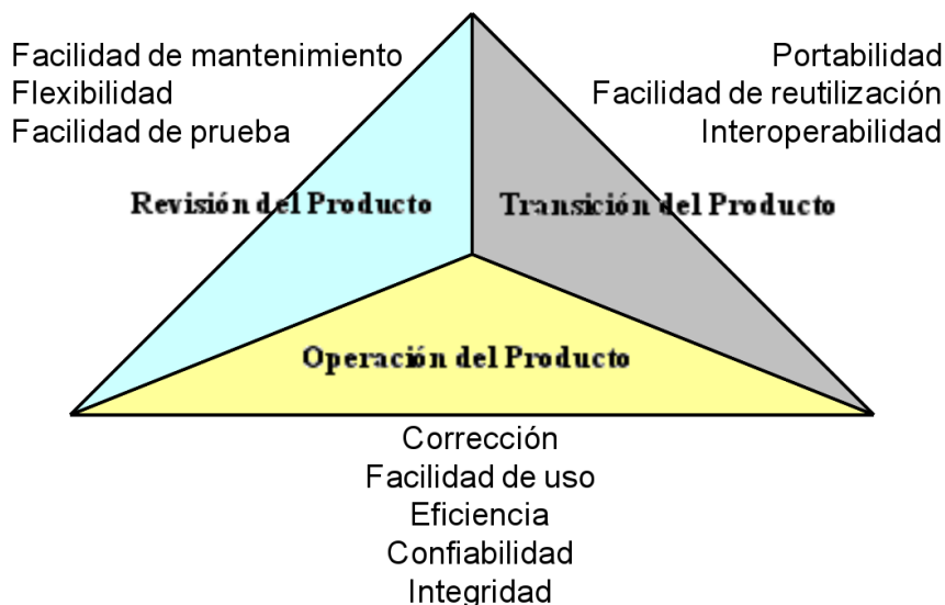
Figura 3.2: Factores de calidad de McCall.
